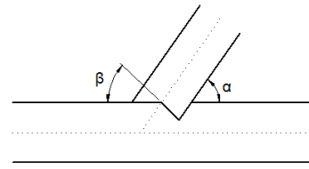
Embrèvement arrière
