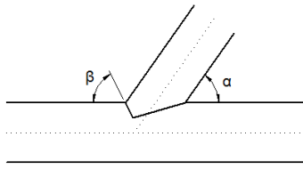
Embrèvement simple
